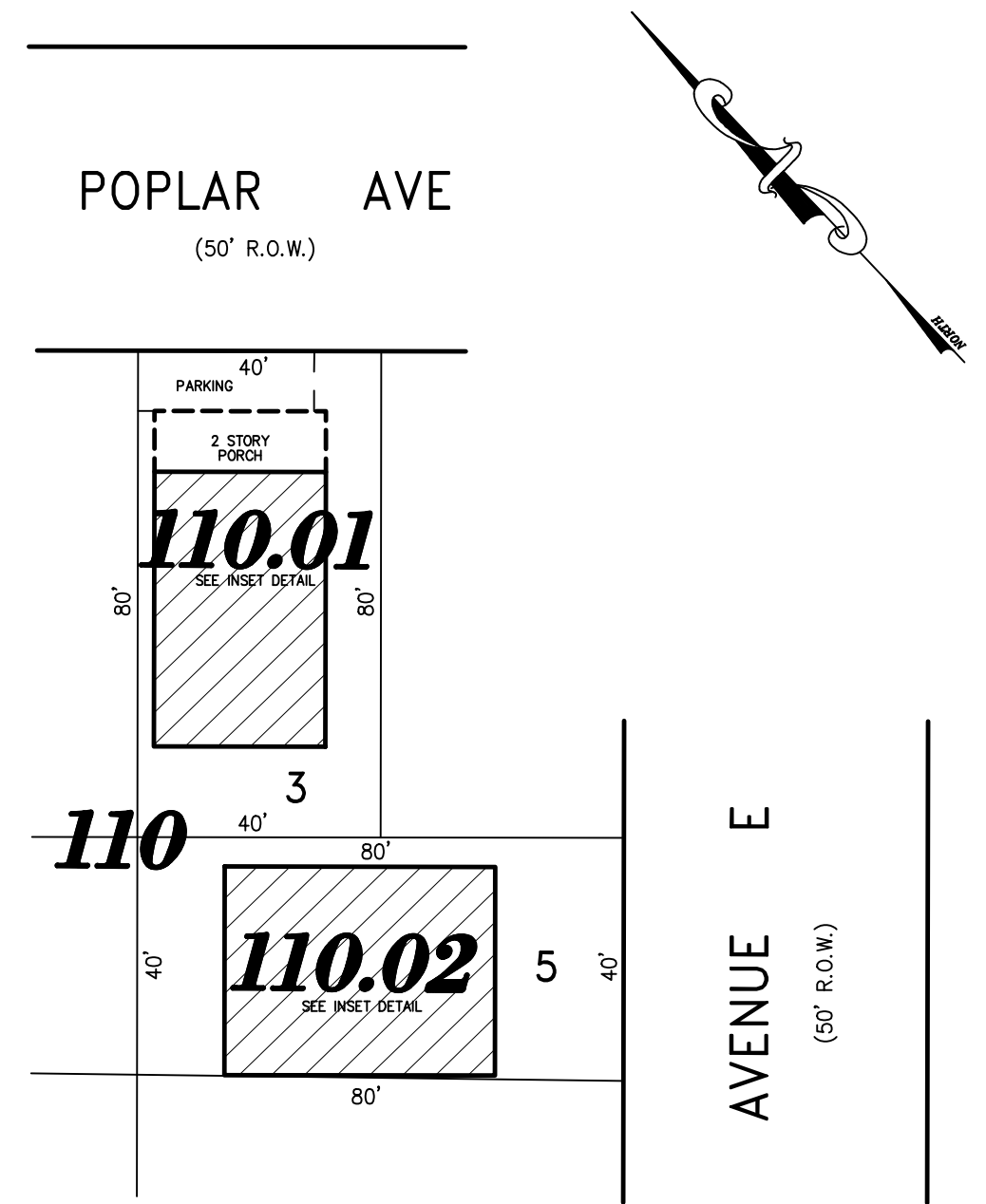
PLAN SCALE: 1"=20'
